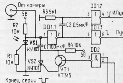
ПРИНЦИПИАЛЬНАЯ СХЕМА БЛОКА ФОРМИРОВАНИЯ ВЫХОДНЫХ ИМПУЛЬСОВ: DD1.1 K155ЛВ8, ОП1-А0У103
